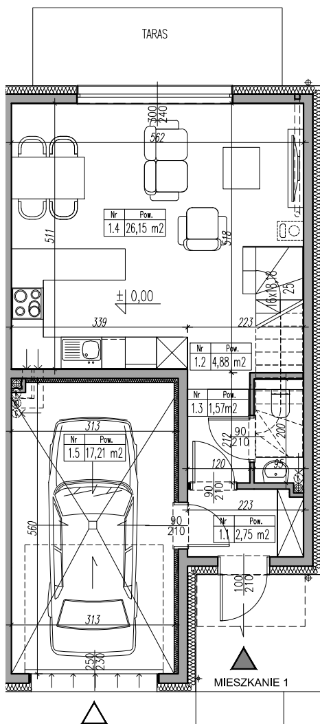
RZUT PARTERU
