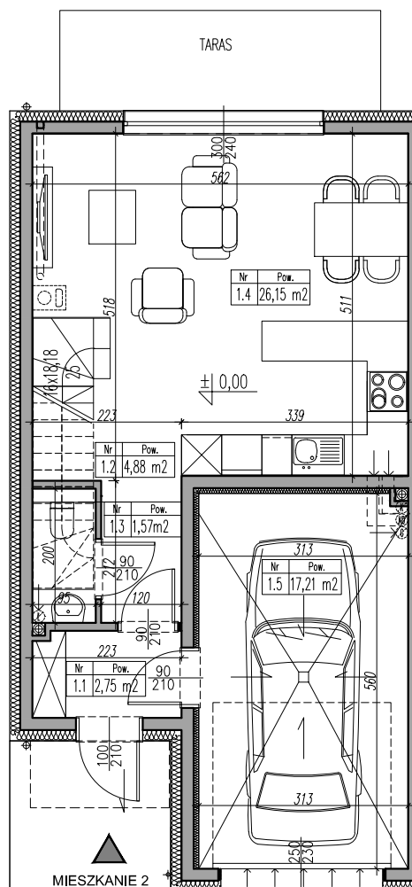
MIESZKANIE 2
