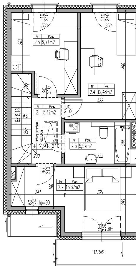
RZUT PIĘTRA
