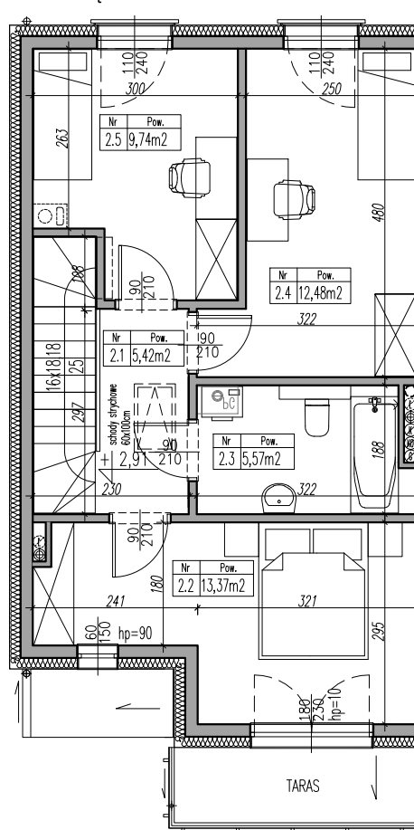
RZUT PIĘTRA
