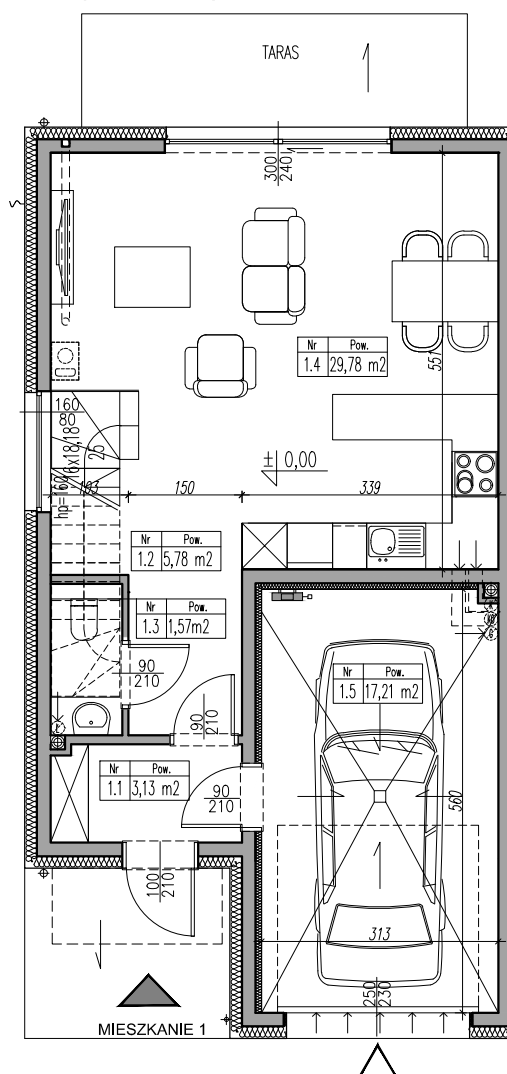
RZUT PARTERU
